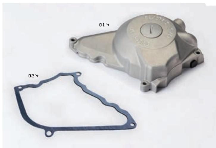
CARTER D'ALLUMAGE POUR DÉMARREUR ÉLECTRIQUE IGNITION COVER ELECTRIC START
